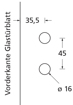
Bohrschema 3-teiliges Glastürband
