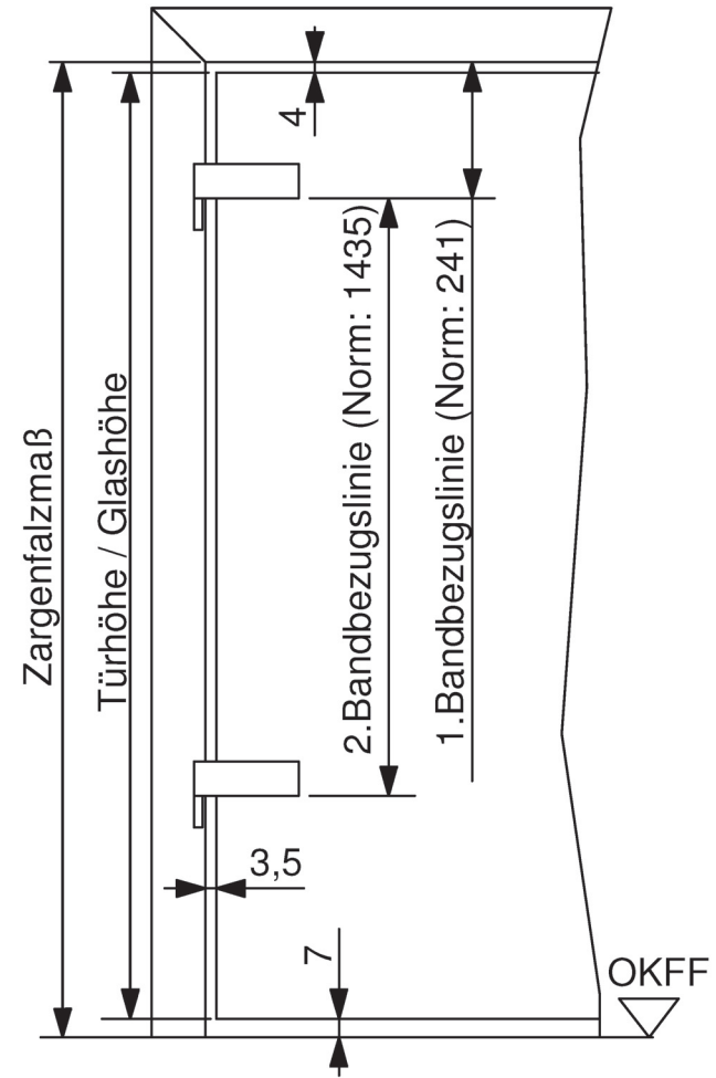
Einbausituation
