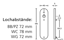
Kurzschildgarnitur 46x180 mm
