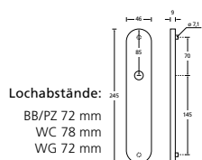
Langschildgarnitur 46x245 mm
