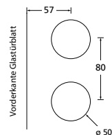
Bohrmaße Office Schloss
