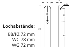
Langschildgarnitur schmal 36x245 mm
