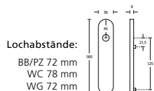
Kurzschildgarnitur schmal 36x180 mm
