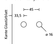
Bohrmaße 2-teiliges Band
