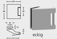
eckig massiv
